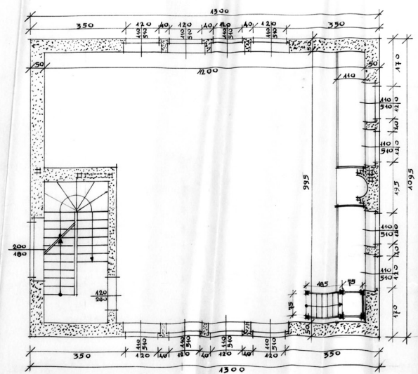
TLOCRT DŽAMIJE
