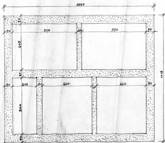
TLOCRT TEMELJA
