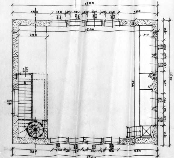
TLOCRT DŽAMIJE
