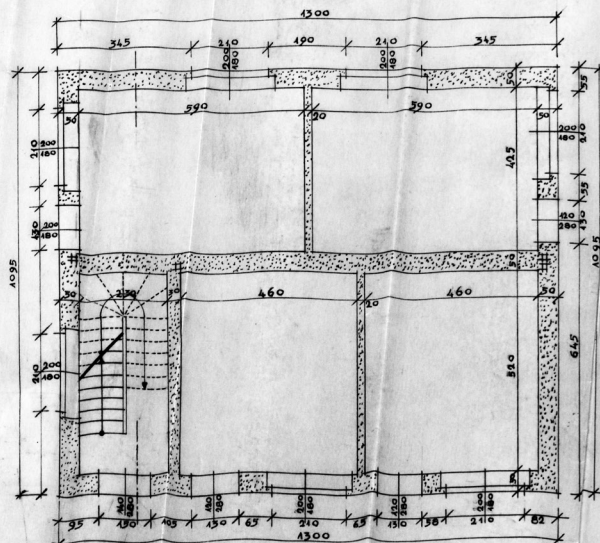
TLOCRT PRIZEMLJA
